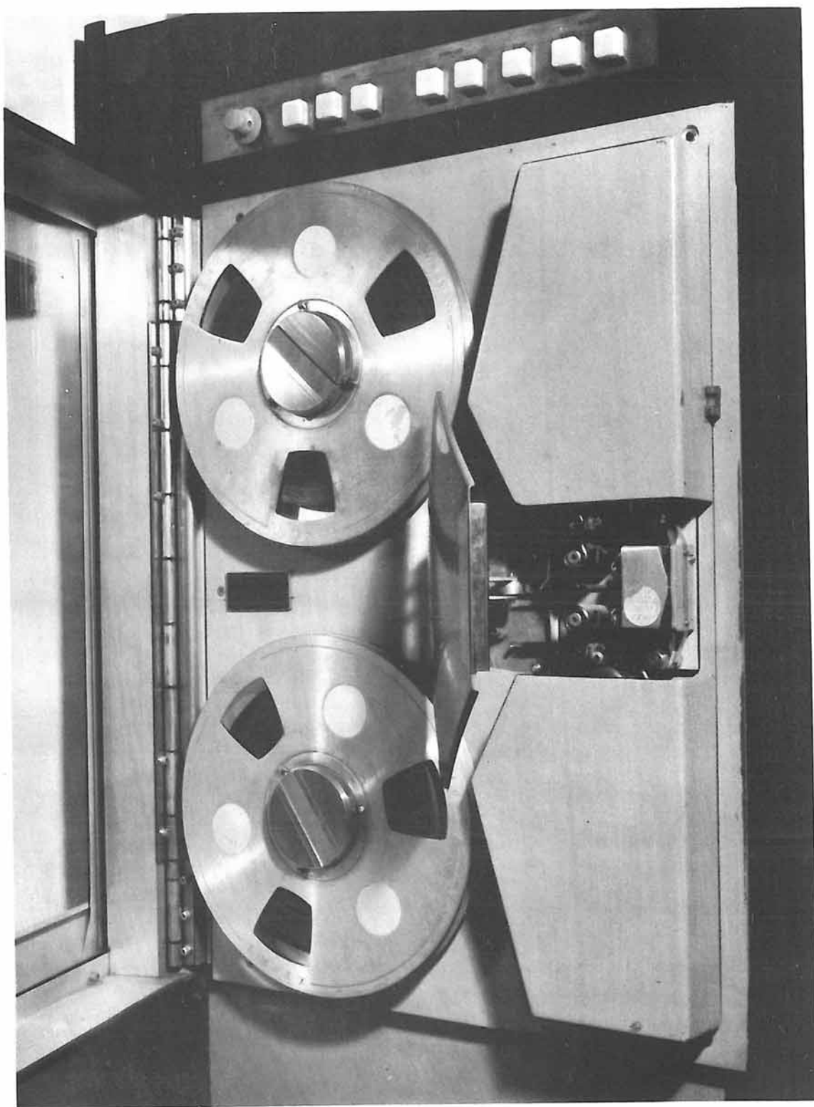
UNITA' A NASTRO MAGNETICO FR-400 ..
